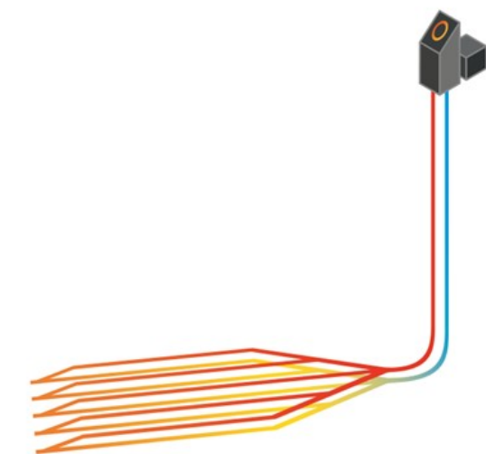
Abbildung: Funktionsweise und Technologie des Eavor-Loop™; Copyright Eavor
