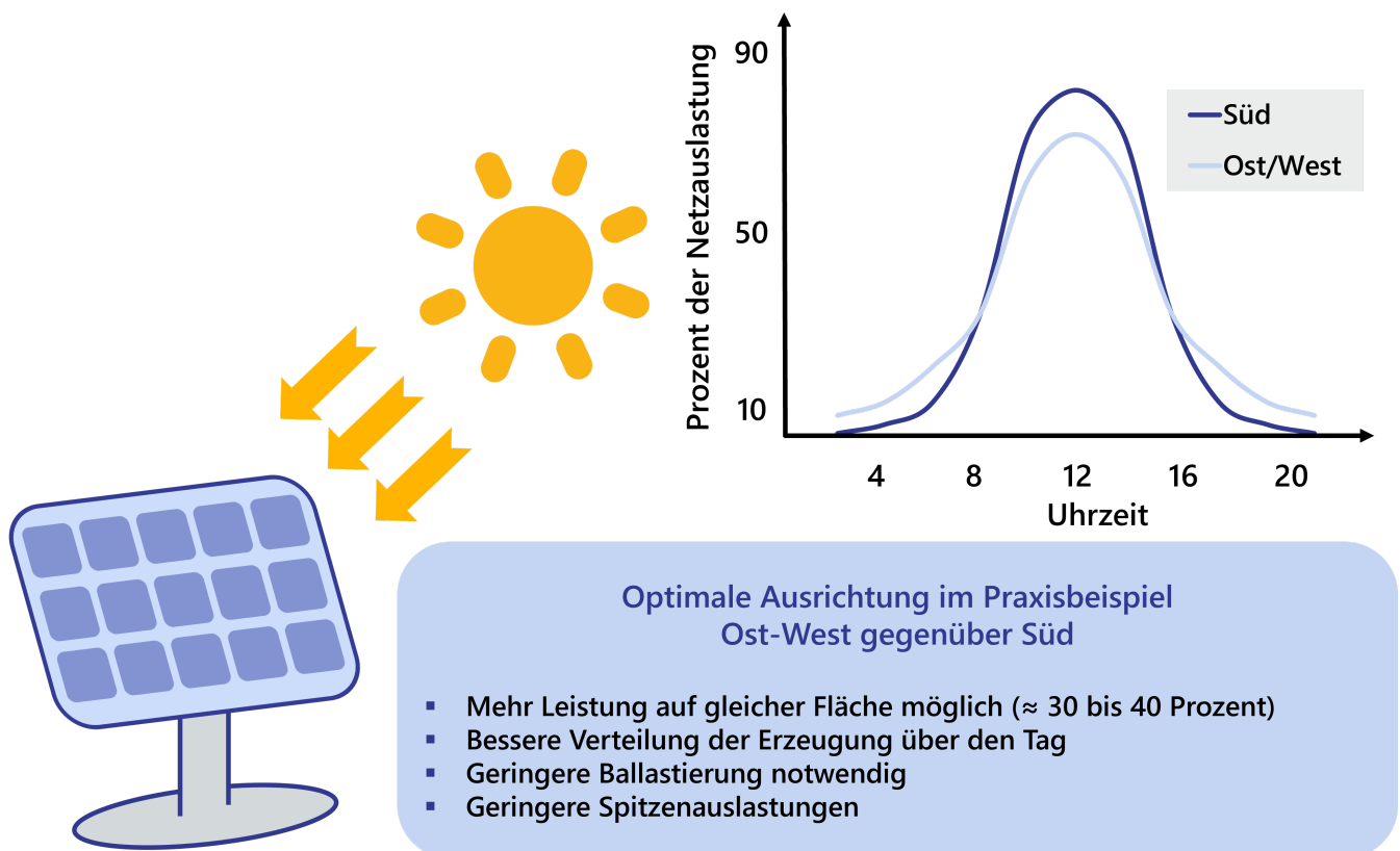
Abbildung 2: Optimale Energieerzeugung durch am Verbrauch orientierte Ausrichtung
