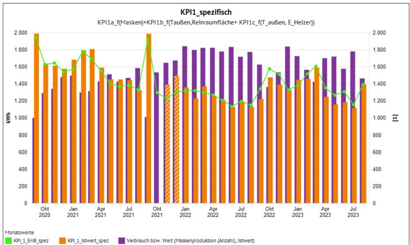
Grafik 3: Key Performance Indicator (KPI) für den spezifischen Energieverbrauch pro Maskenunit
